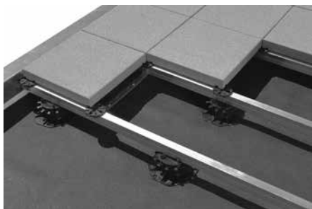
Verlegebeispiel
