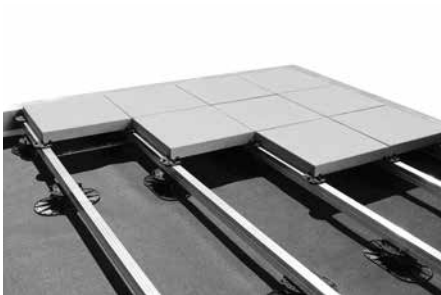
Verlegebeispiel
