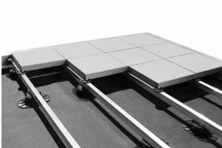
Verlegebeispiel
