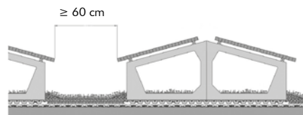
Solaraufständerung „Sattel“
