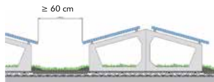
Solaraufständerung „Sattel“
