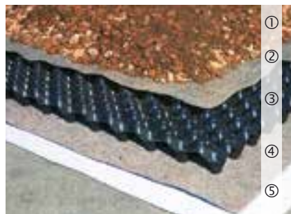
Systemaufbau „Lavendelheide“
