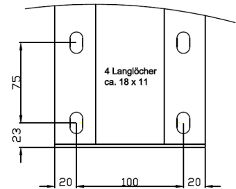
Lochbild des Schraubflansches der Geländerbasis GB
